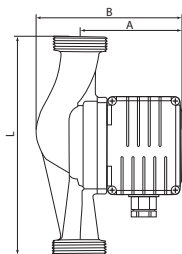
Wymiary instalacyjne
