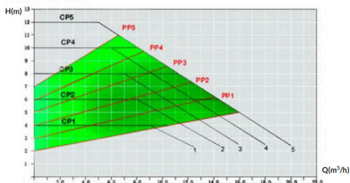
NOVA MAX 50-12/250
