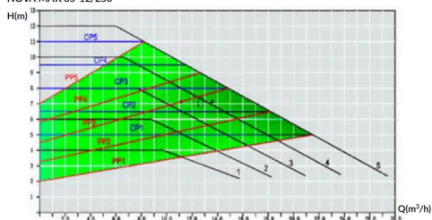
NOVA MAX 65-12/250
