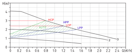
IVO 25-40/180
