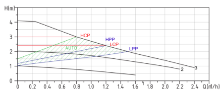
IVO 25-40/180
