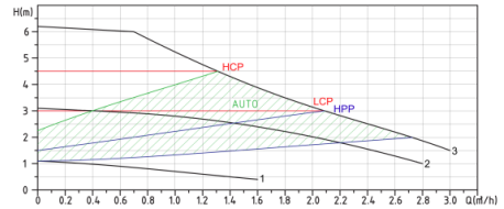
IVO 25-60/180 (130)
