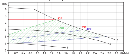
IVO 25-60/180 (130)
